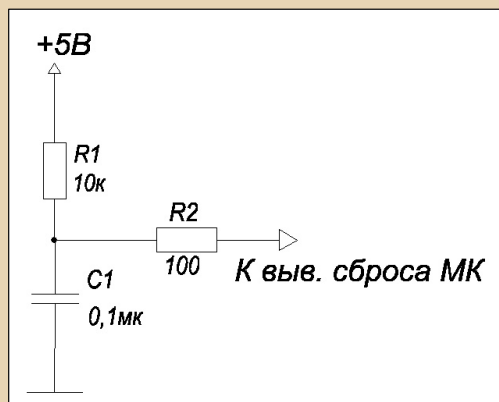
Рис. 2. Схема сброса с RC-цепочкой от частотомера Д. Богомолова
