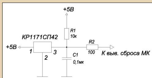
Рис. 3. Схема сброса с использованием КР1171СП42
